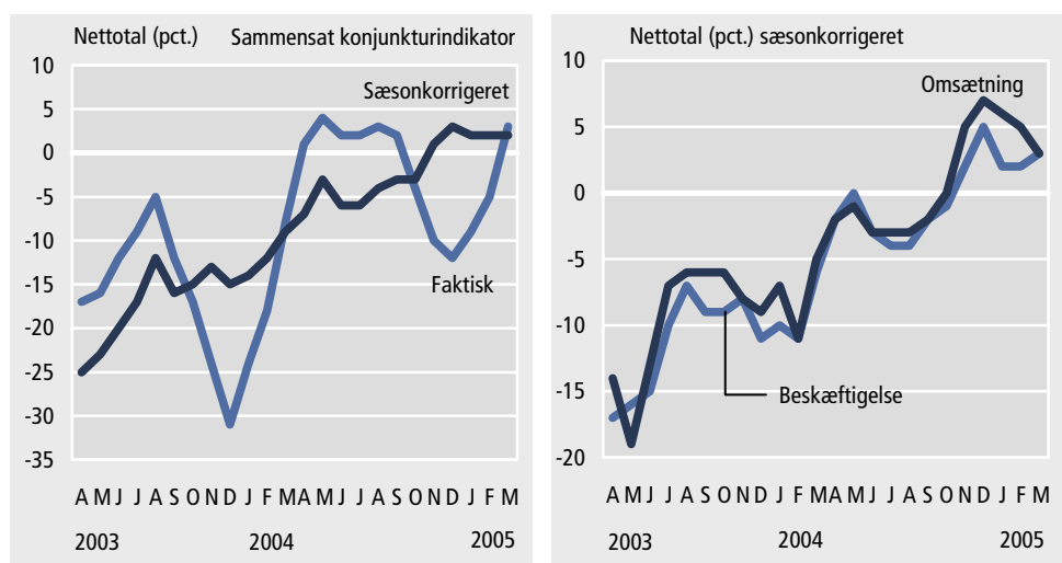
Figur 1. Sammensat konjunkturindikator for bygge og anlæg og forventninger til beskæftigelse og omsætning. Marts - maj 2005
