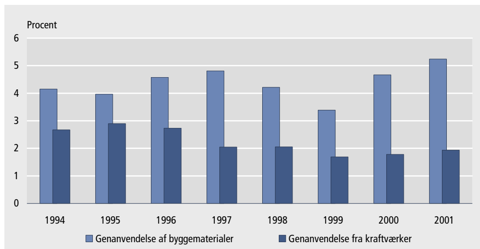
Figur 8. Genanvendelse af byggematerialer i pct. af tilsvarende indvundne råstoffer
