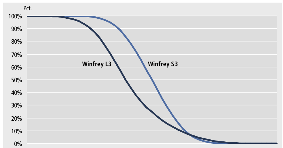
Figur 1. Overlevelseshedsfunktioner
