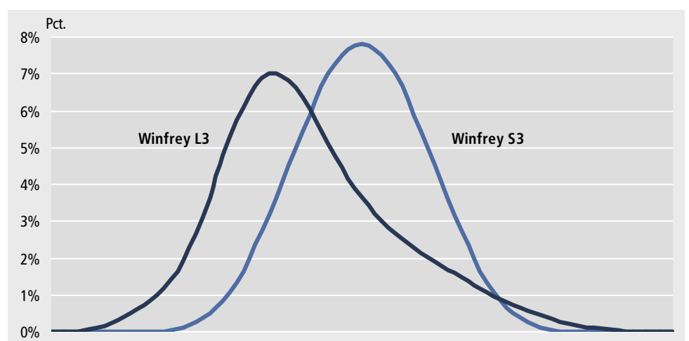
Figur 2. Tæthedsfunktioner
