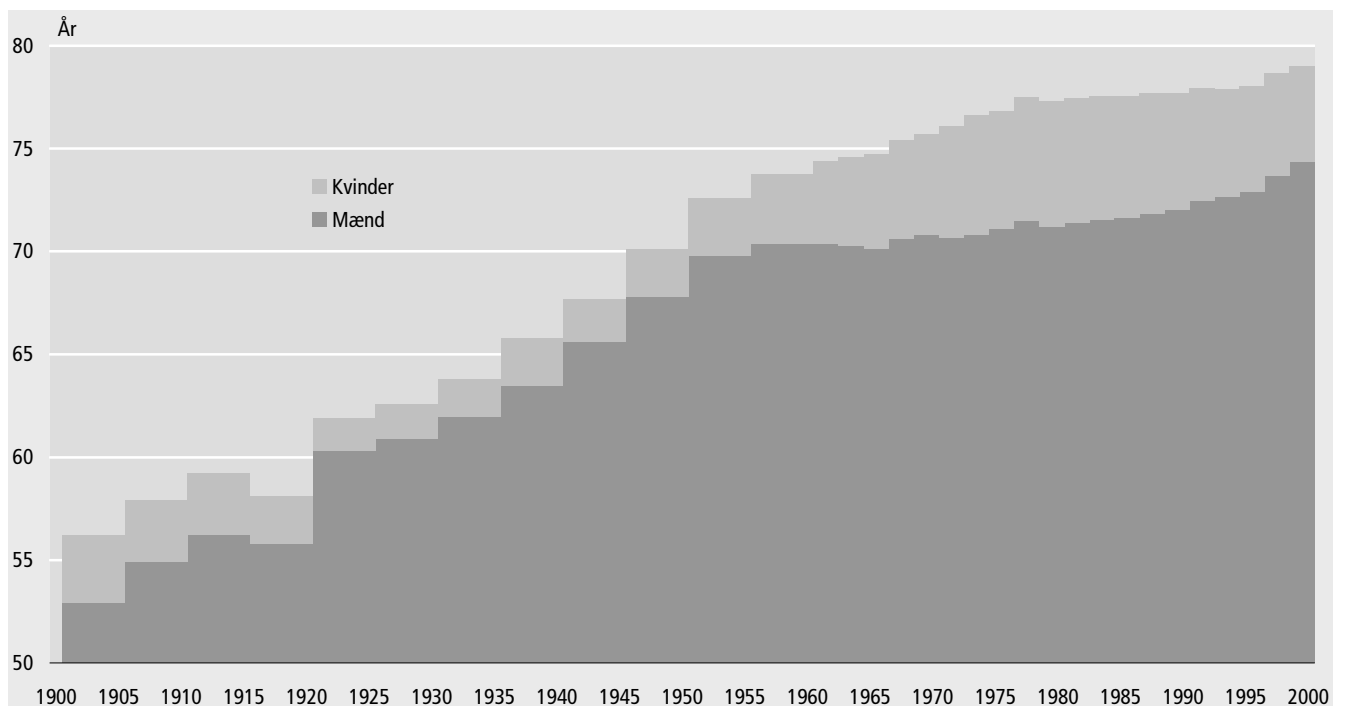
Figur 12. Middellevetid 1901-2000 Life expectancy 1901-2000
