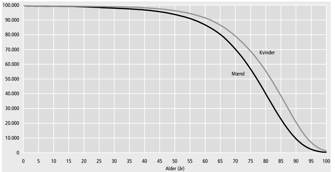
Figur 11. Overlevelseskurve for mænd og kvinder 1999/2000 Survivors in life table for 1999/2000
