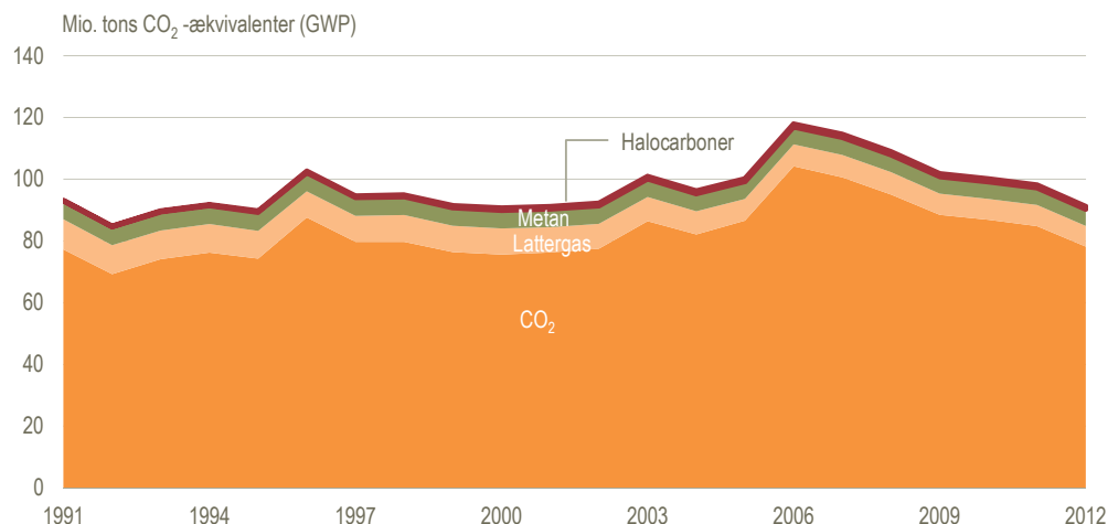
Figur 4 Udledning af drivhusgasser fra danske økonomiske aktiviteter
