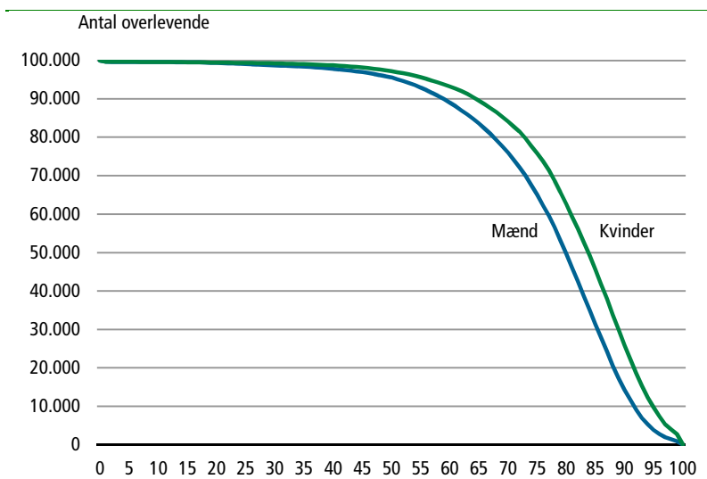
Figur 4.1 Overlevelseskurve for mænd og kvinder. 2009/2010 Survivors in life table. 2009/2010
