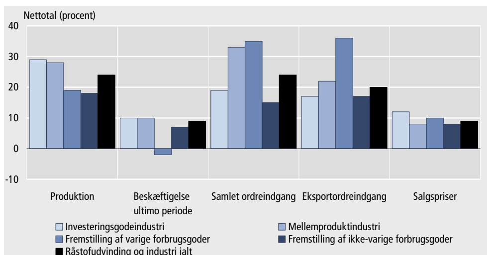
Figur 2. Industriens forventninger til 2. kvrt. 2004 i forhold til 1. kvrt. 2004
