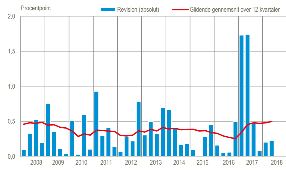
Figur 2. Revision (absolut)
