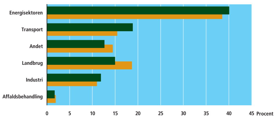
Figur 3 Udledning af drivhusgasser (GWP) fordelt på sektorer
