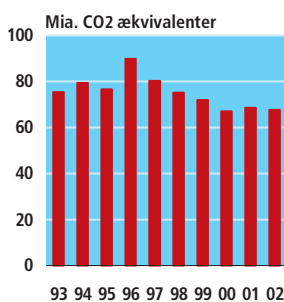
Figur 2 Udslip af drivhusgasser 1993-2002
