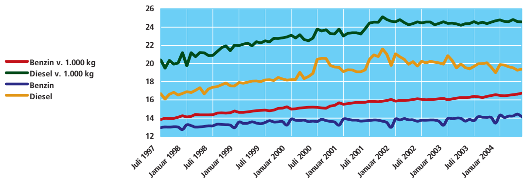
Figur 5 Energieffektiviteten for nyregistrerede personbiler 1998-2004
