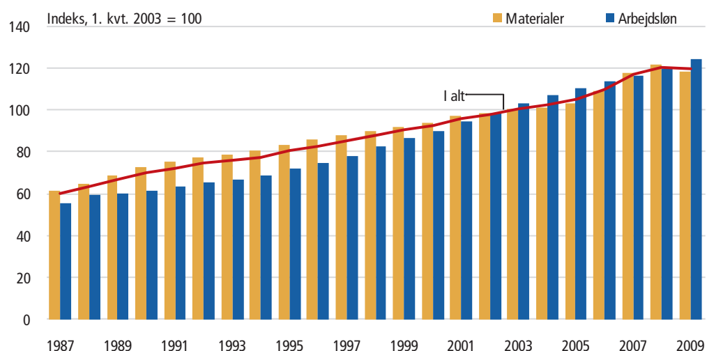
Figur 7 Byggeomkostningsindeks for boliger
