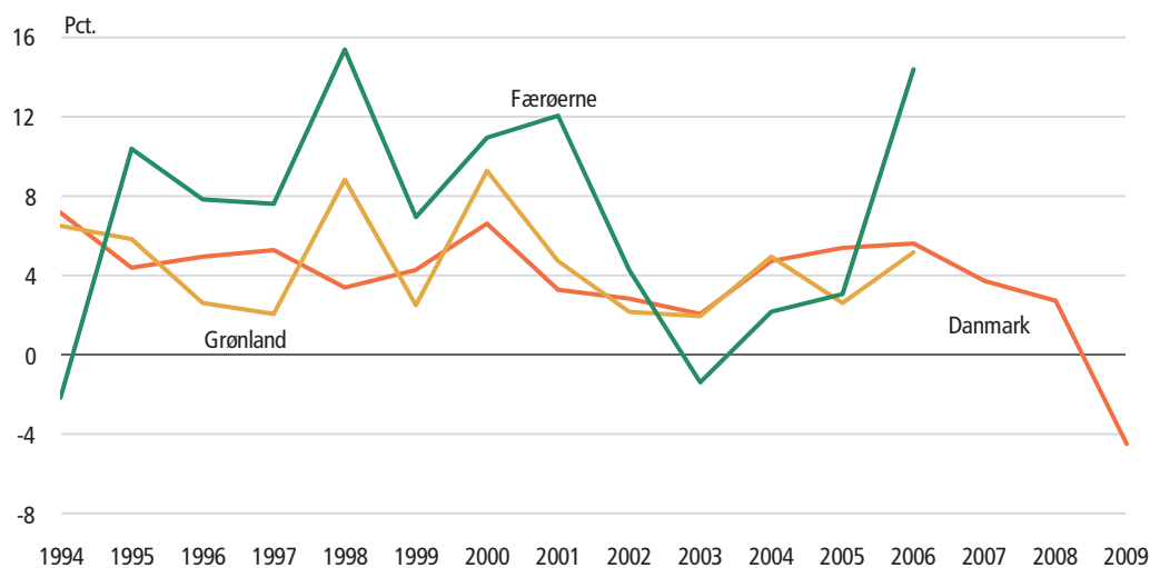
Figur 4 Udviklingen i BNP i årets priser
