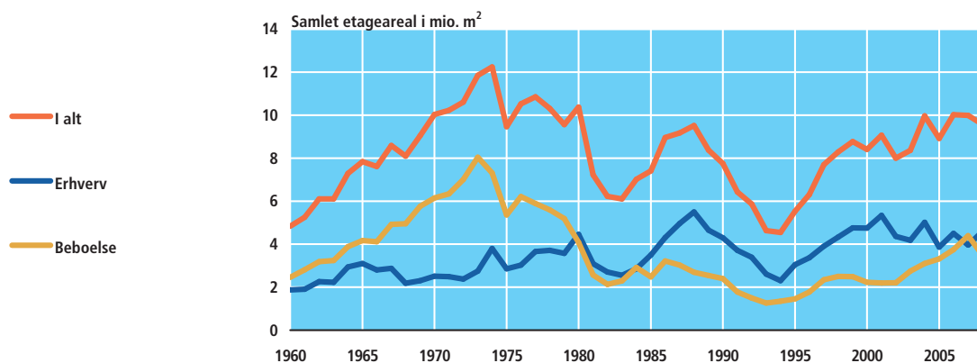
Figur 5 Fuldført byggeri, samlet etageareal
